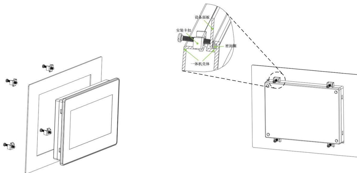
图 3.3-10 固定配件安装示意图
