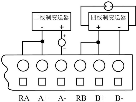
图 2.2-27 二线制、四线制电流输入接线图例
