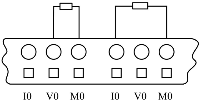
图 2.2-33 CPU 模拟量输出接线图
