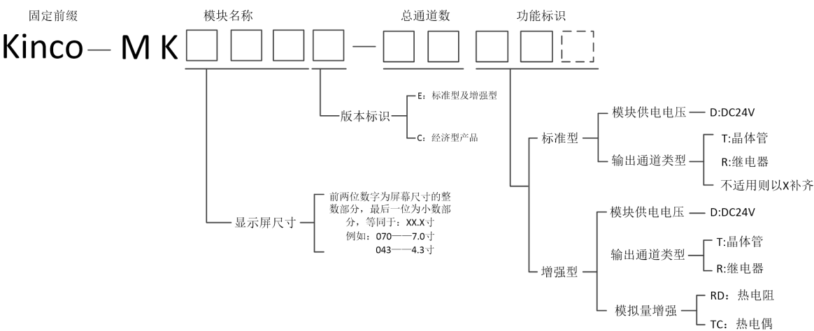
图 1.2-1 MK 系列命名规则示意
