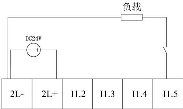
图 2.2-25 源型输入（DI）接线方式
