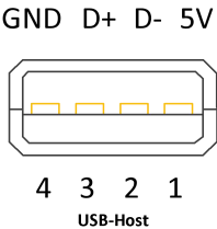
图 2.2-7 USB-Host 接口引脚
