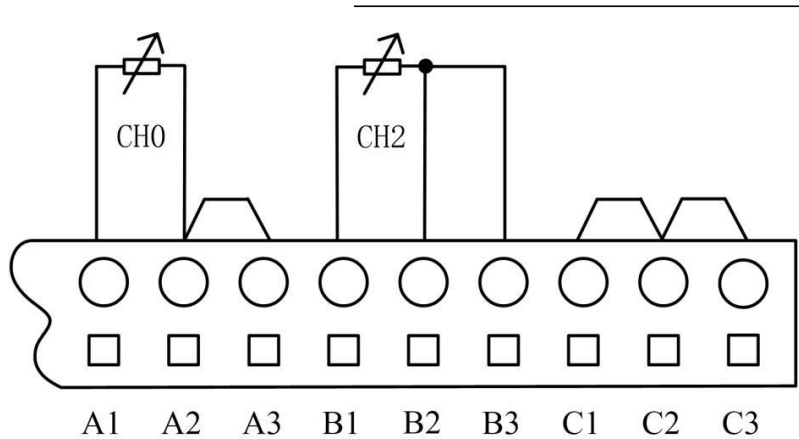
图 2.2-30 模拟量输入短接示意
