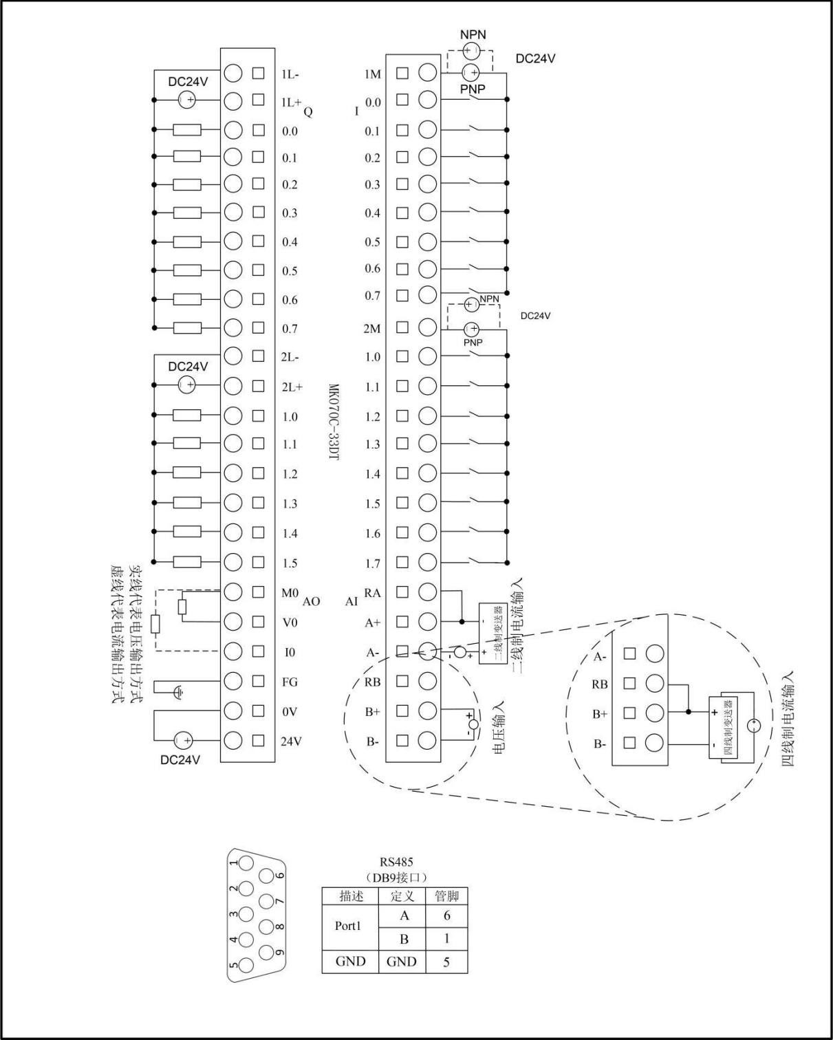
图 2.2-41 MK070C-33DT 接线总图
