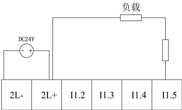
2.2-26 漏型输出（DO）接线方式
