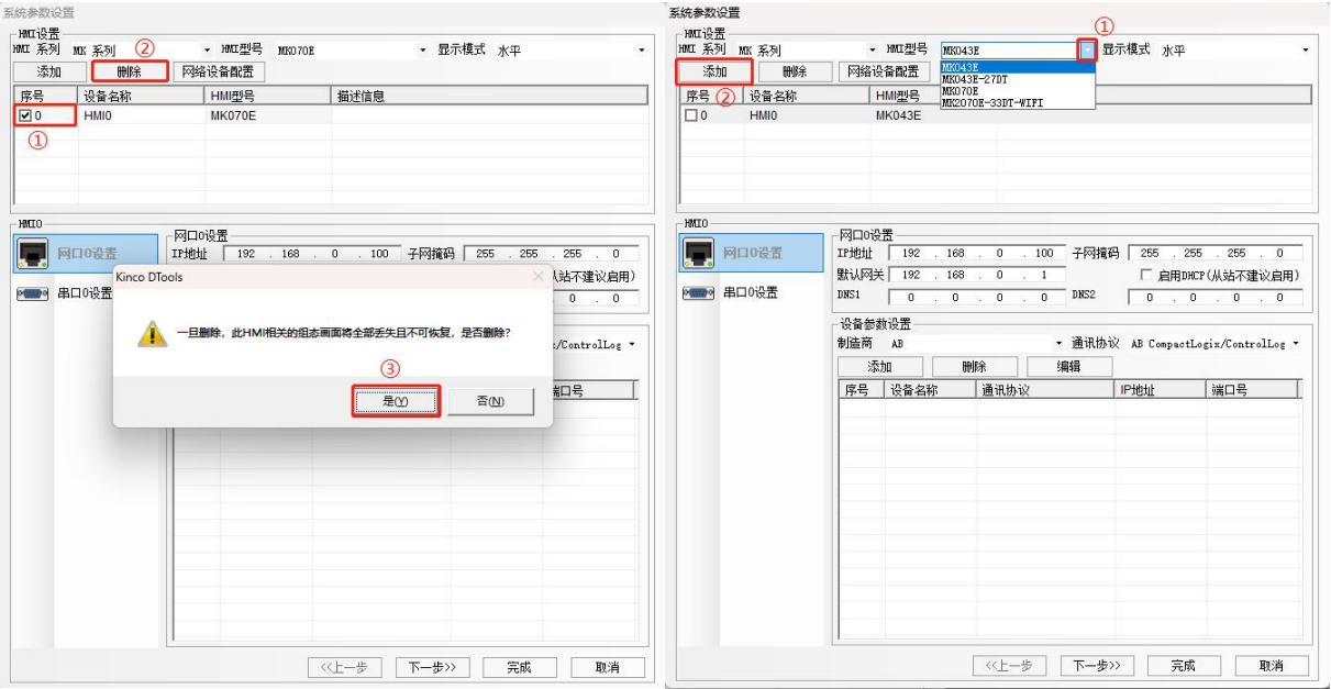
图 5.2-3 修改 HMI 型号步骤
