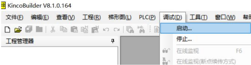
图 2.2-3 切换 PLC 状态
