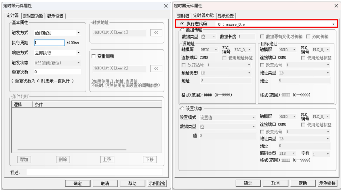
图 5.5-6 定时器元件执行宏文件设置
