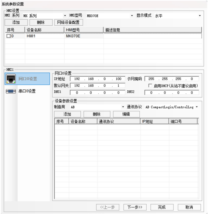
图 5.2-2 系统参数设置界面
