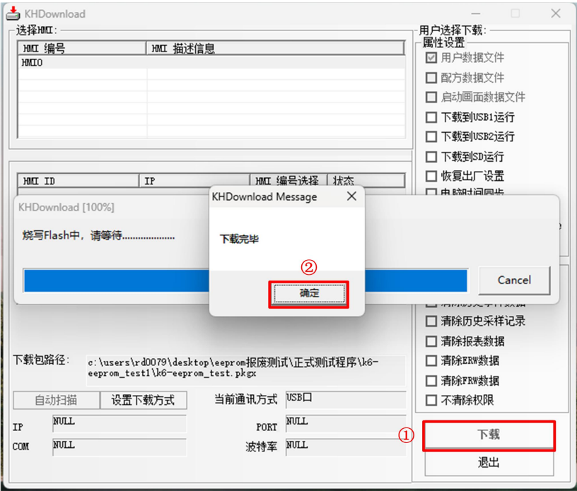
图 5.10-4 下载工程操作步骤 2
