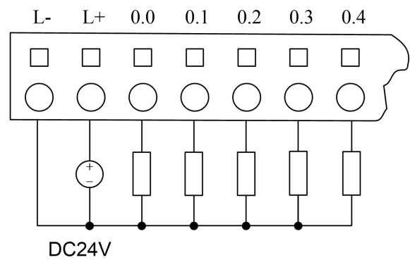
图 2.2-22 晶体管型 DO 接线图例
