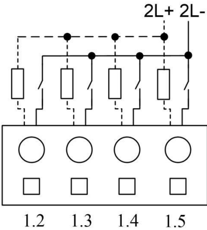
图 2.2-24 DIO 通道接线图例
