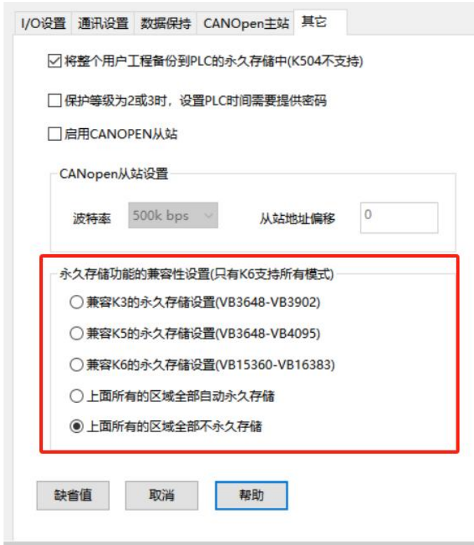
图 2.2-13 永久存储设置
