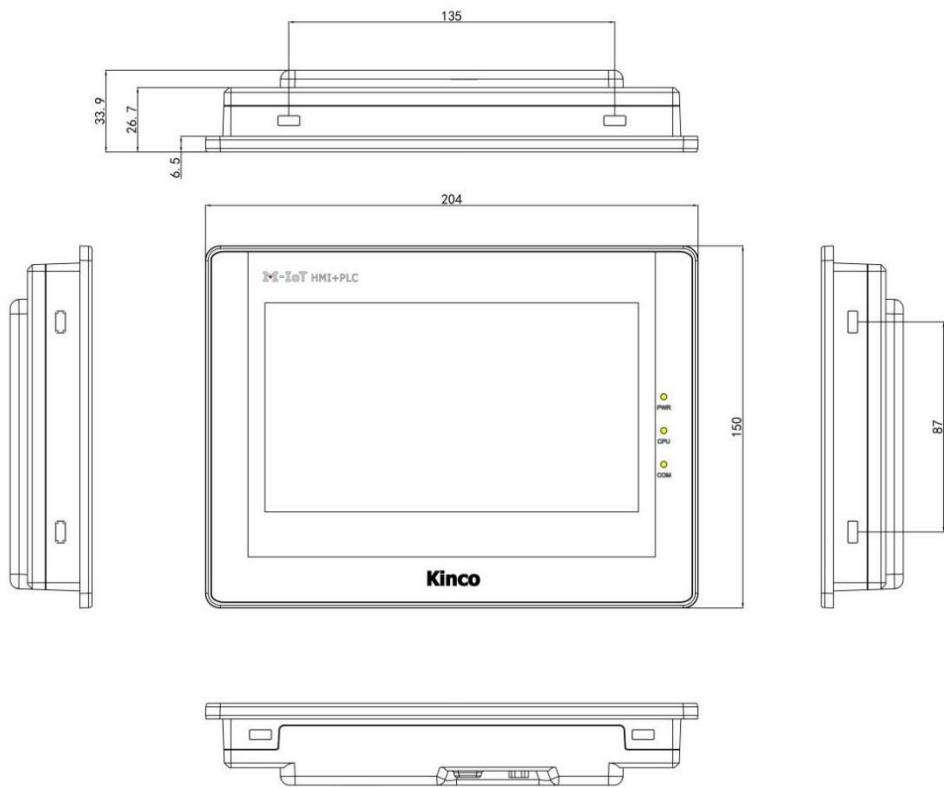
图 2.2-43 MK070E-33DT/MK070E-32DX/MK070E-27DRT/MK070C-33DT 模块尺寸图
