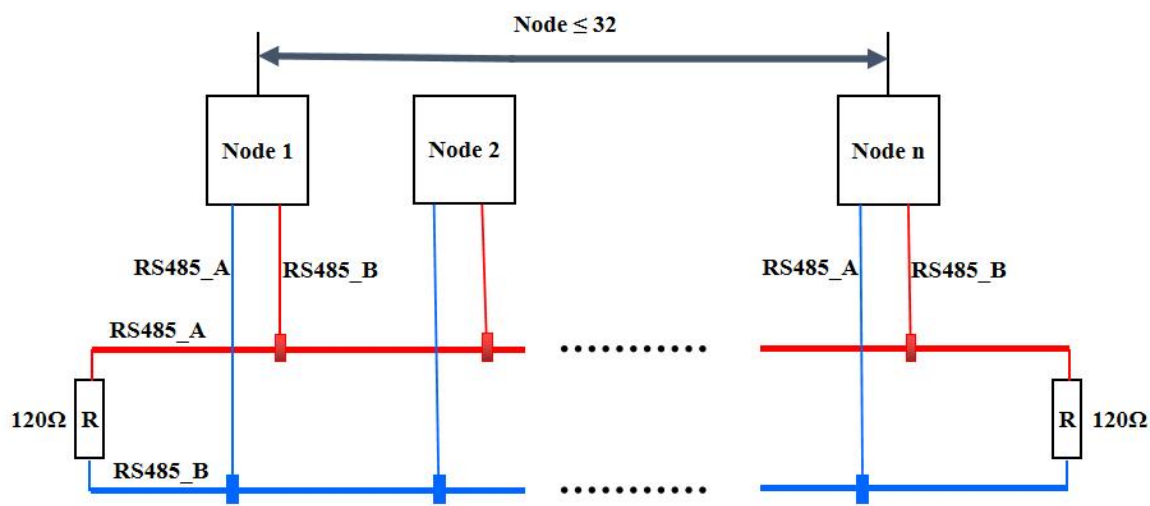
图 2.2-6 RS485 拓扑结构
