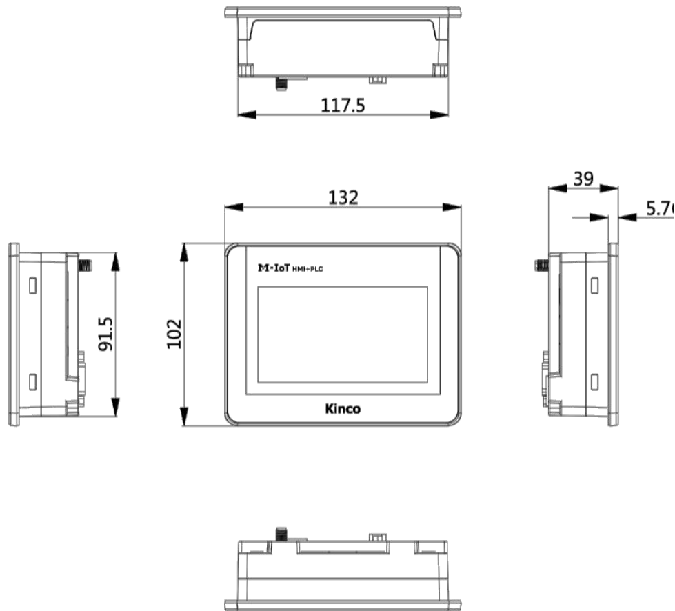
图 2.2-45 MK043E-27DT 模块尺寸图
