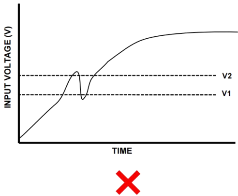
图 3-13 非单调性电源
