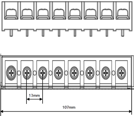
图 3-5 FD145 驱动器 X5 接口尺寸图
