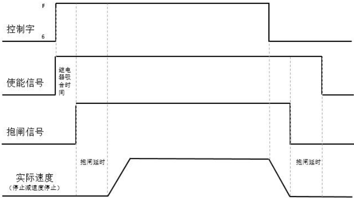
图 5-8 快速停止模式为 2 时电机抱闸时序
