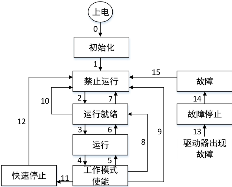
图 5 - 2 DS402 状态机
