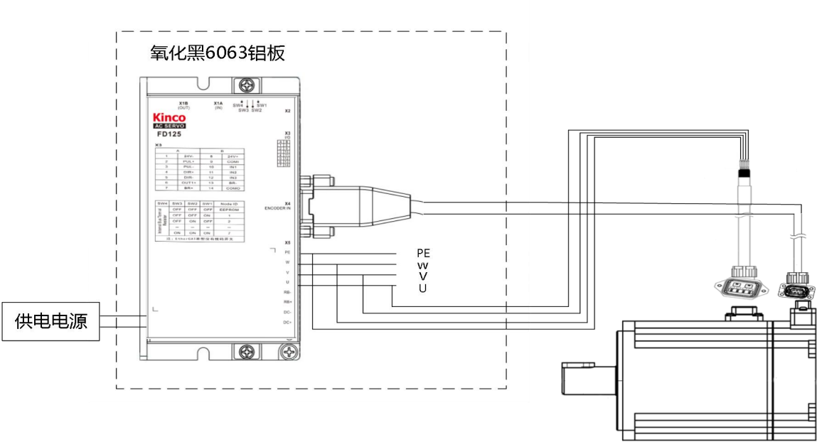
图 2-1 辅助散热安装图
