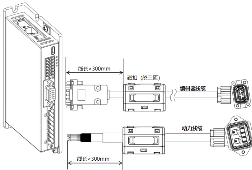
图 3-11 磁环安装图
