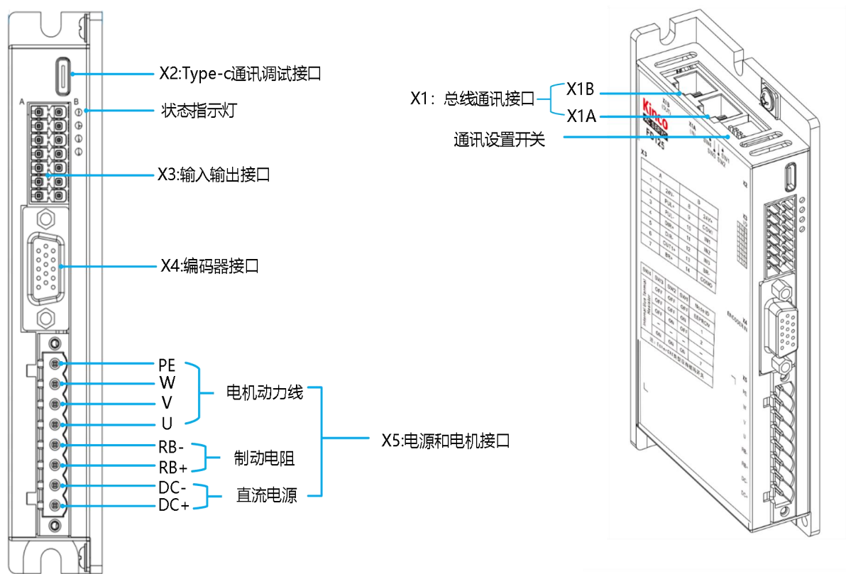
图 3-1 FD1X5 系列各部分名称
