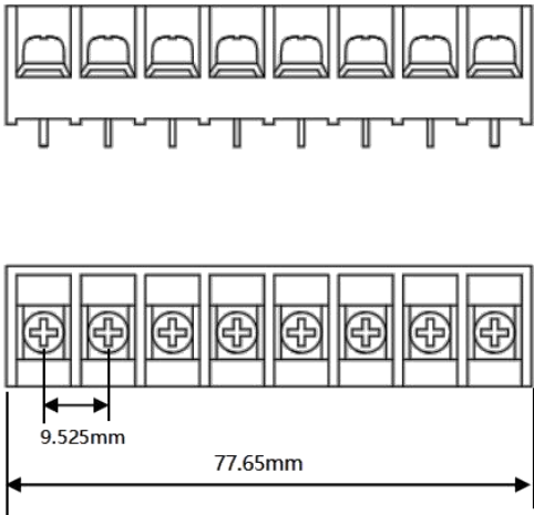
图 3-4 FD135 驱动器 X5 接口尺寸图
