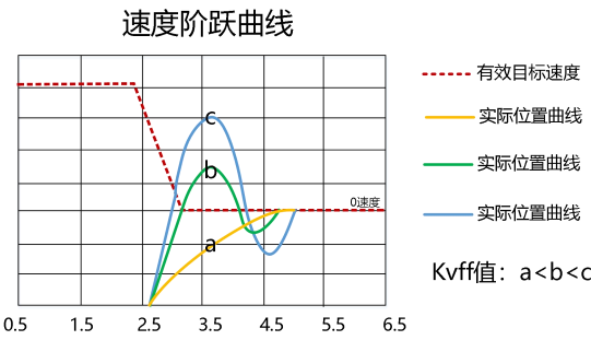
图 6-4 位置环比例增益调节后的速度阶跃曲线
