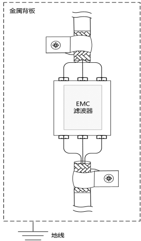
图 3-8 EMC 噪音滤波器安装示意图
