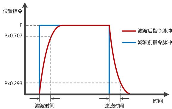
图 5 - 6 脉冲滤波说明
