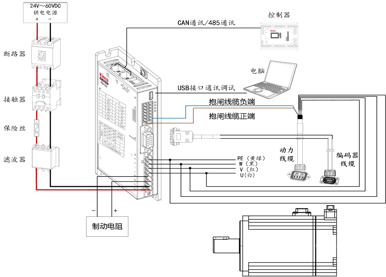
图 3-2 FD1X5 系列外部接线图
