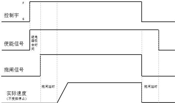
图 5-7 快速停止模式为 0 时电机抱闸时序
