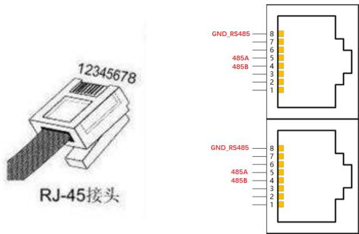
图 8 - 1 FD1X5 的 RS485 接口及定义
