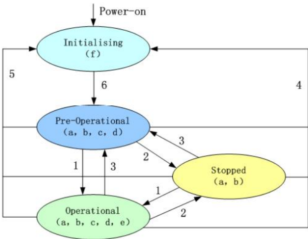
图 9-6 节点状态转换图
