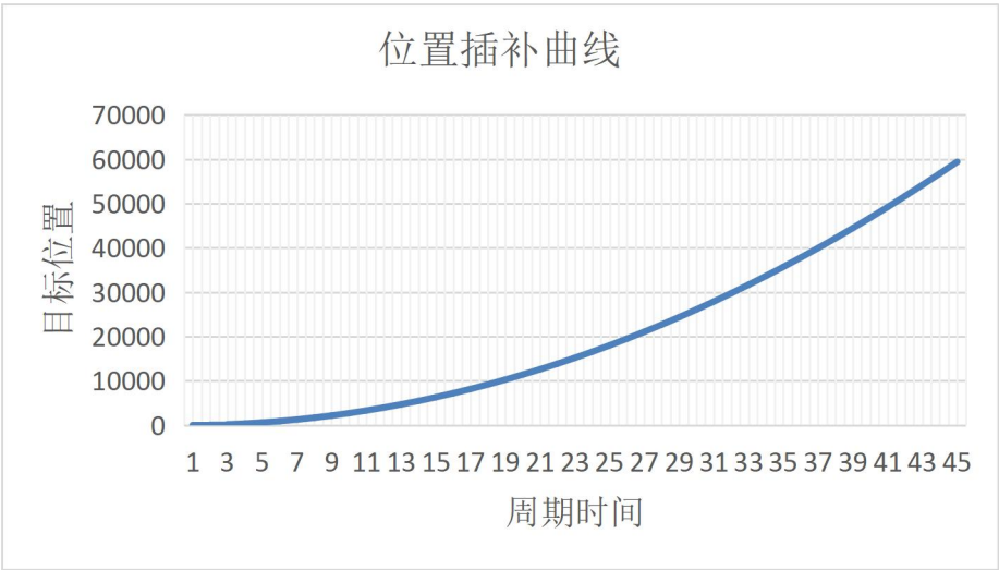
图 9-7 位置插补曲线
