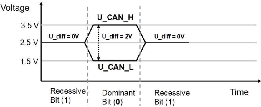
图 9-1 CAN 信号标识
