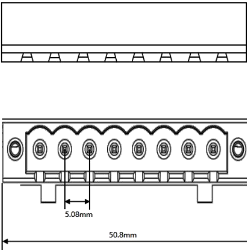
图 3-3 FD125 驱动器 X5 接口尺寸图
