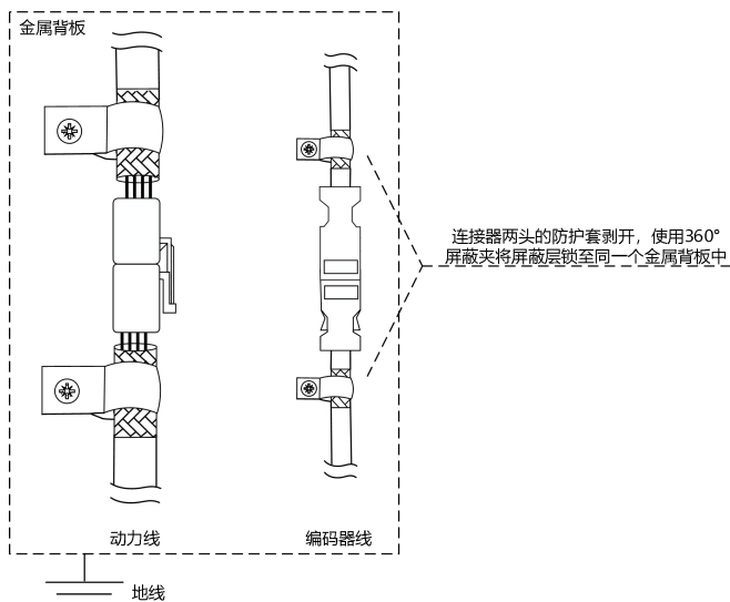
图 3-10 FD1X5 驱动器连接器侧动力线/编码器线屏蔽层 2*处理方式
