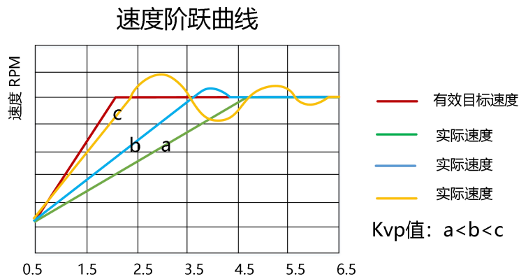
图 6-2 速度环比例增益调节后的速度阶跃曲线
