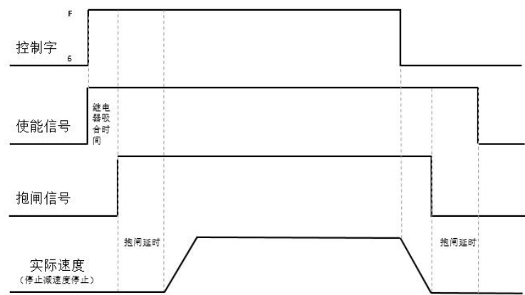
图 5-8 快速停止模式为 2 时电机抱闸时序
