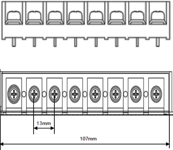
图 3-5 FD145 驱动器 X5 接口尺寸图
